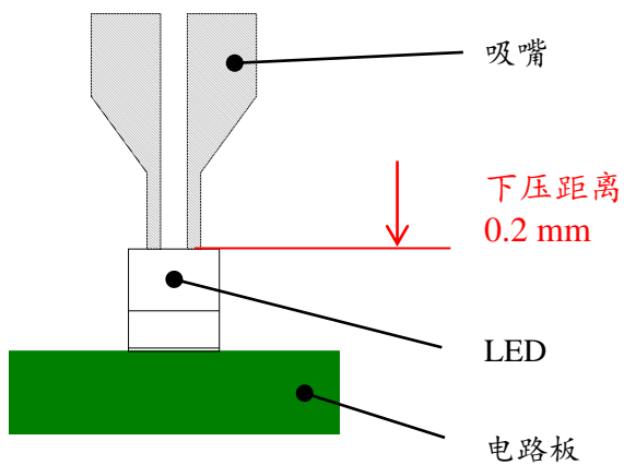
图17. 贴放高度 (日亚推荐)
