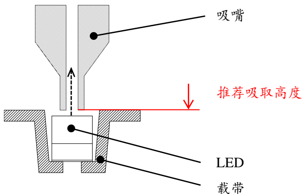
图16. 吸取高度 (日亚推荐)
