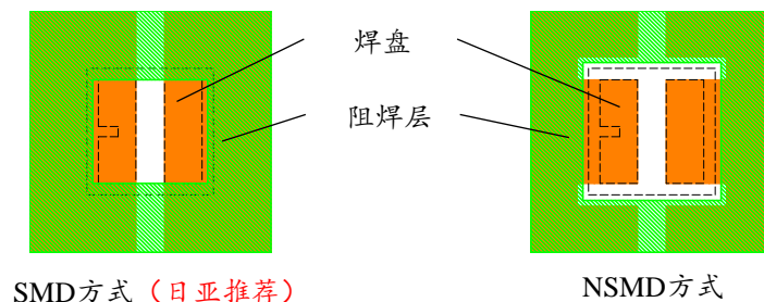
图10. 电路板焊盘图案的形成方法
