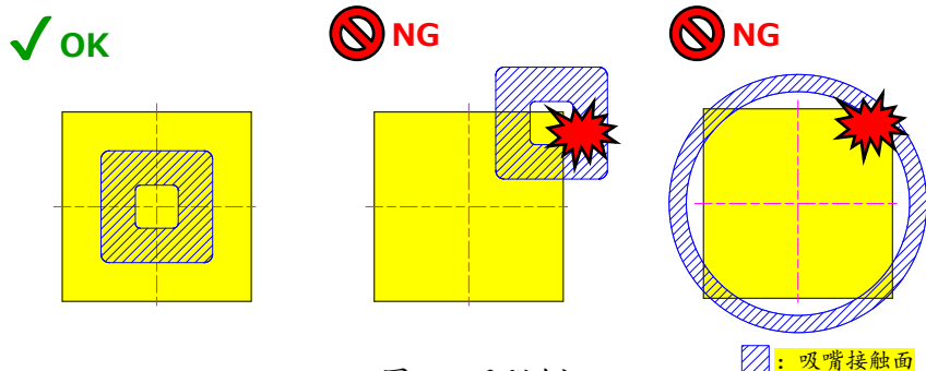
图14. 吸附例
