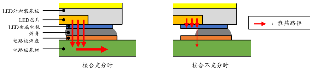
图12. 不同接合状态下的散热
