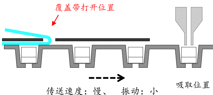
图15. 覆盖带打开位置
